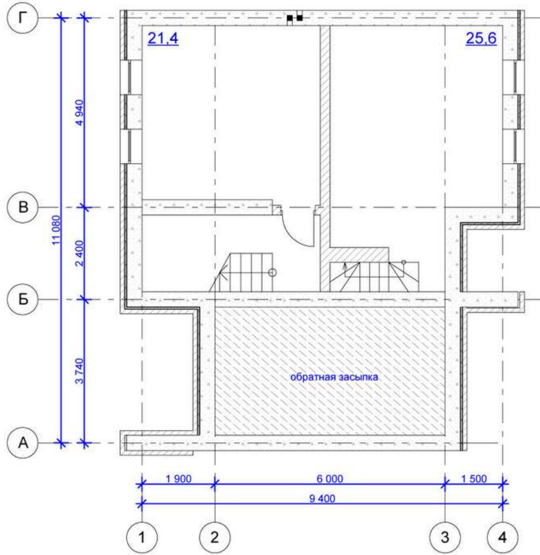
План подвала
