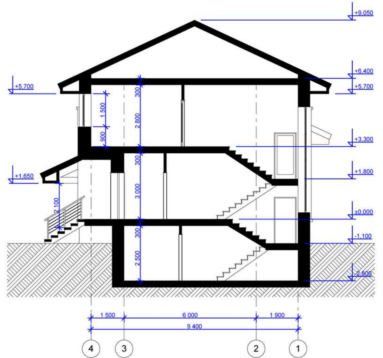
Разрез 1-1
